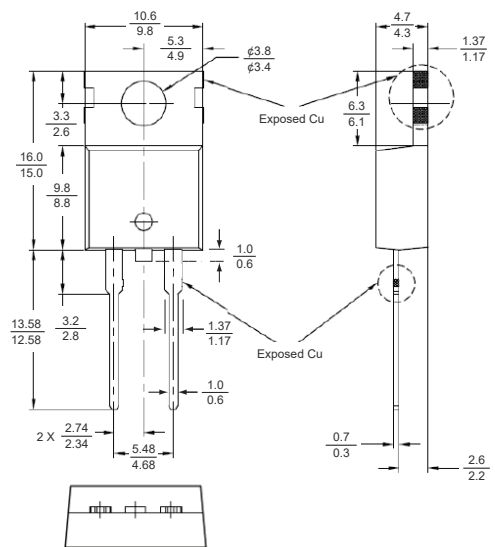
TO-220AC
