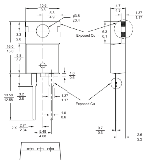
TO-220AC
