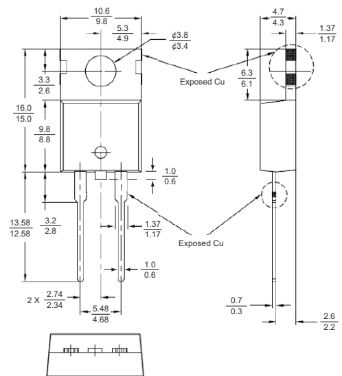
TO-220AC
